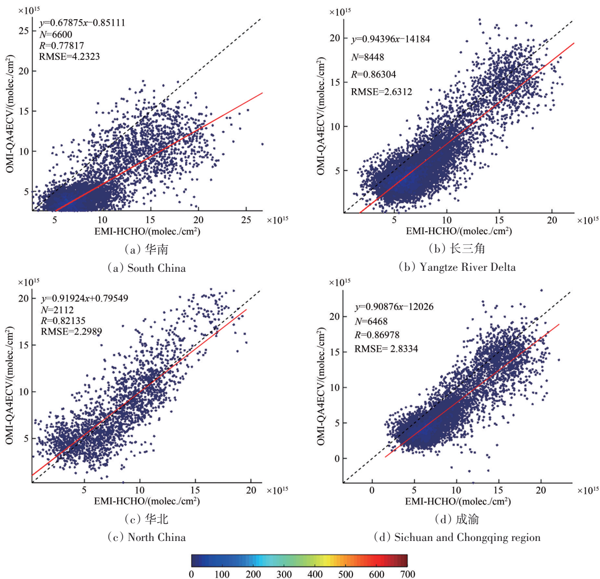
图7 EMI与OMI QA4ECV HCHO交叉对比
