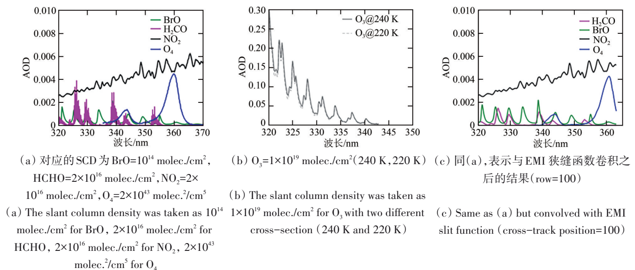
图1 BrO, HCHO, NO 2 , O 4 与O 3 光学厚度 Fig. 1 Optical depth of BrO, HCHO, NO 2 , O 4 and O 3
